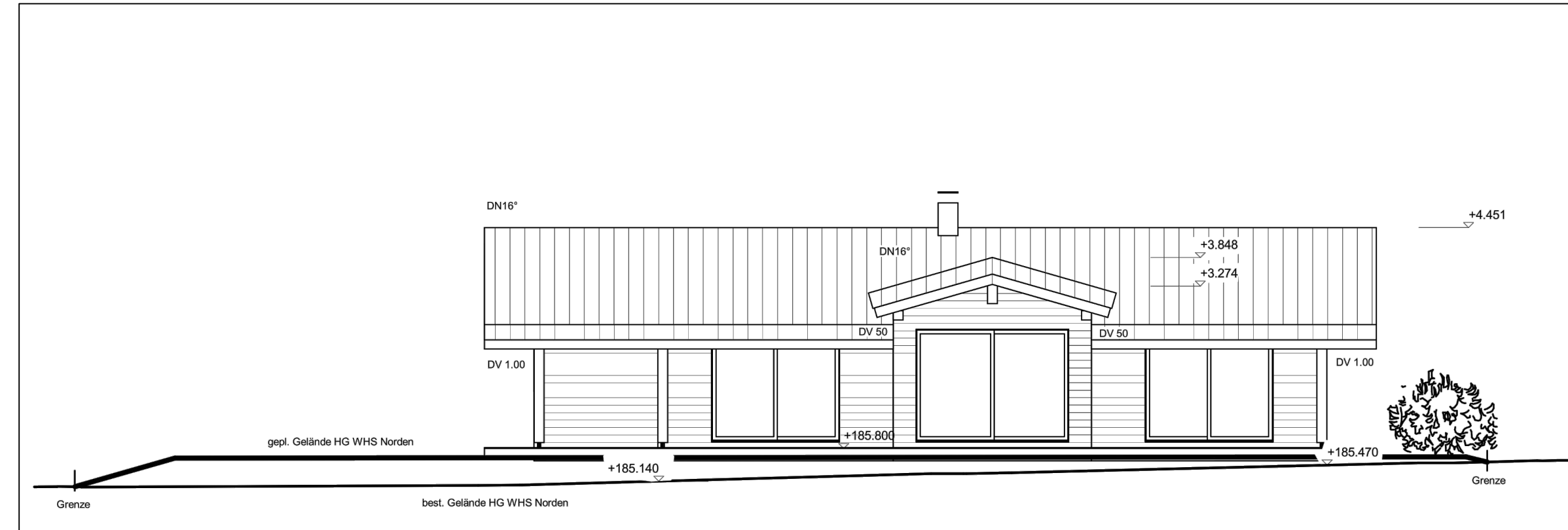
Nord-Ansicht
