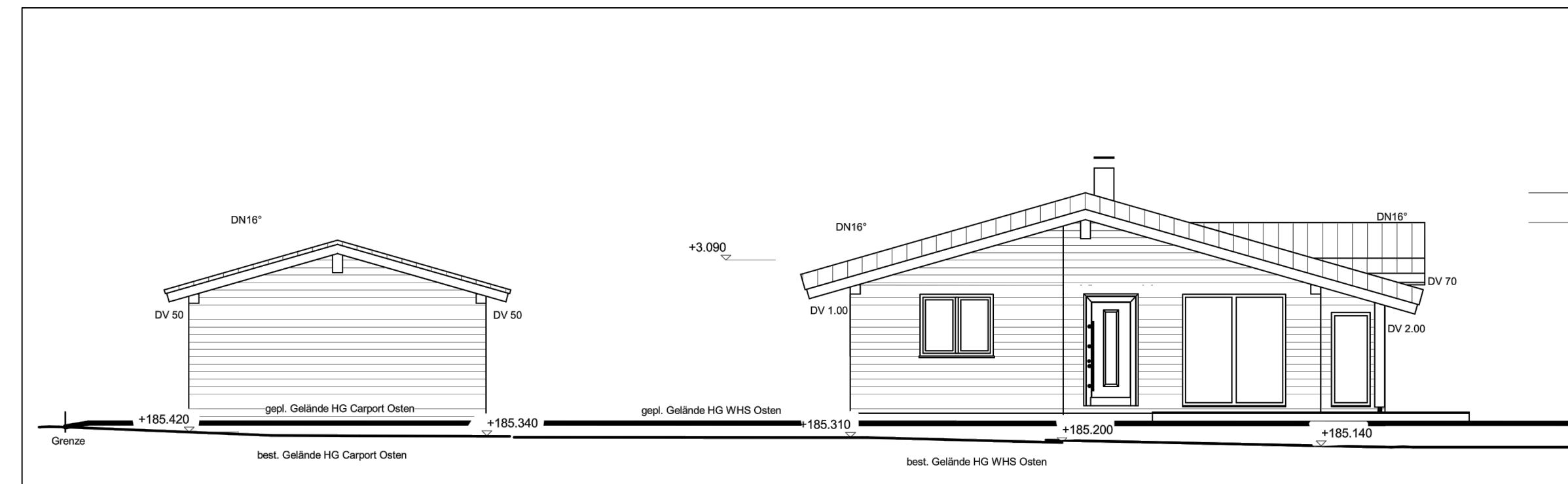
Ost-Ansicht
