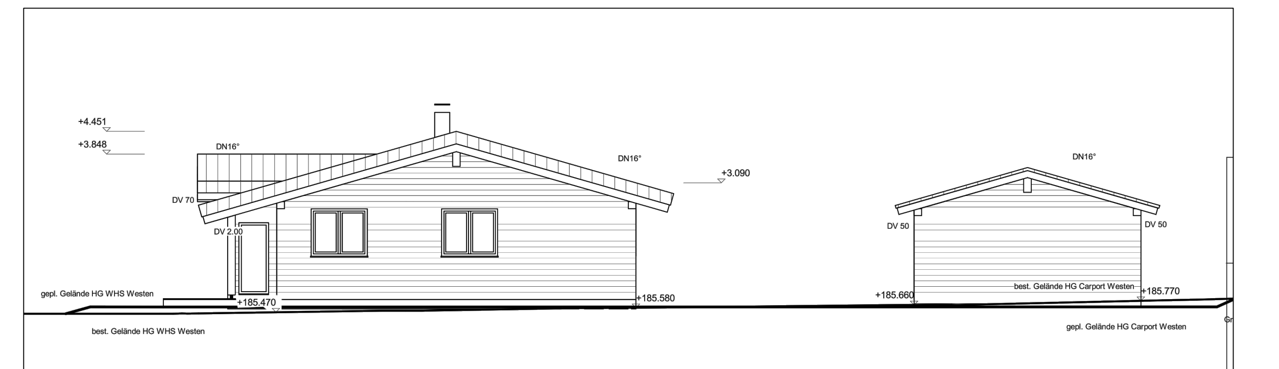
West-Ansicht
