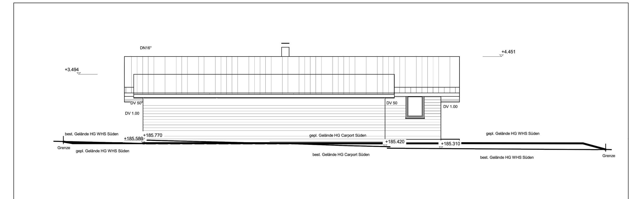
Süd-Ansicht
