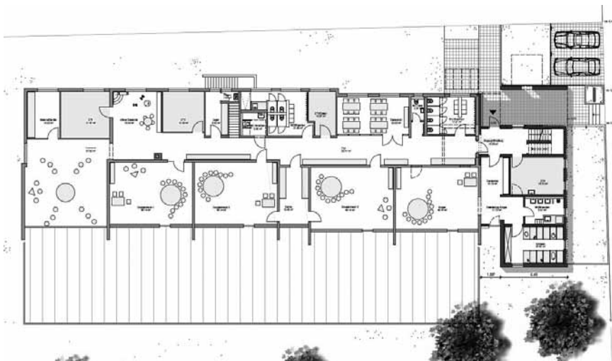
Entwurf Grundriss Erdgeschoss
