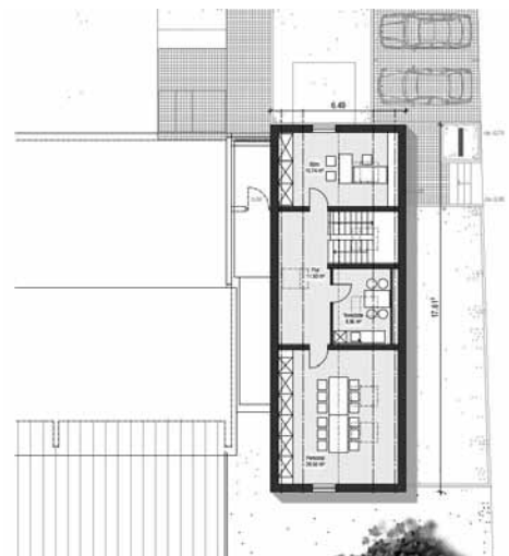
Entwurf Grundriss Obergeschoss (Erweiterung)
